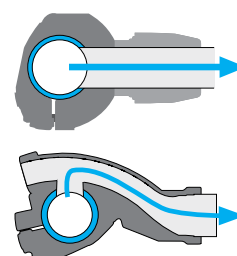
Horizontaler Abgang
