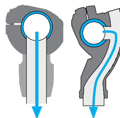
Vertikaler Abgang
