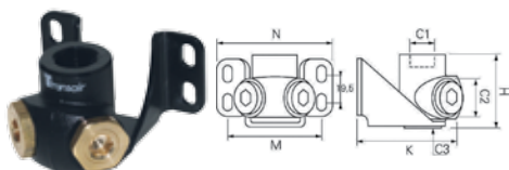
WANDANSCHLUSS MIT 2 AUSGÄNGEN 90° BSP ZYLINDRISCH
